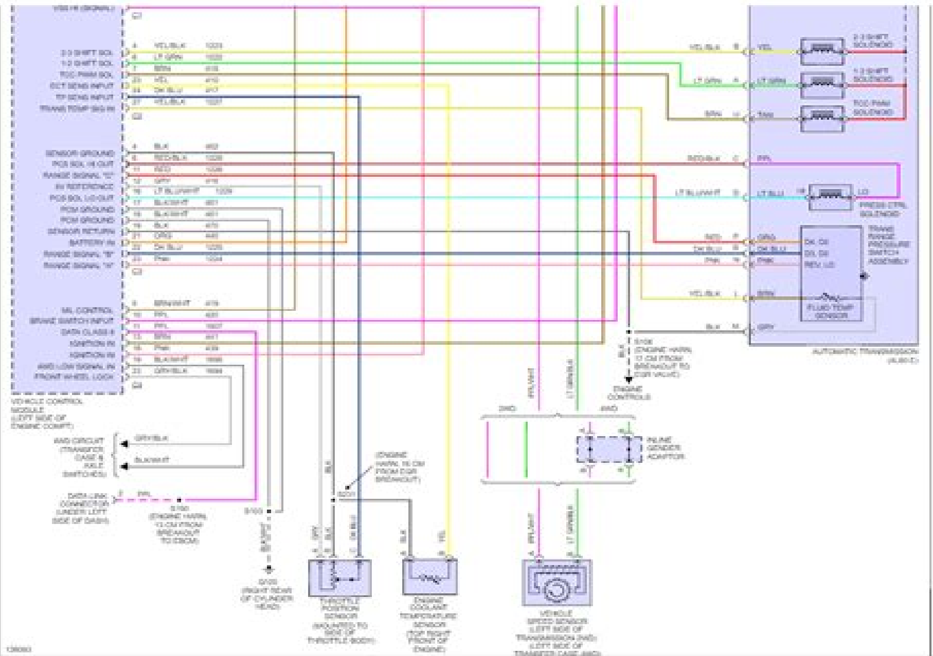
Fig 1: 5.7L VIN K, A/T Circuit, 4L60-E
