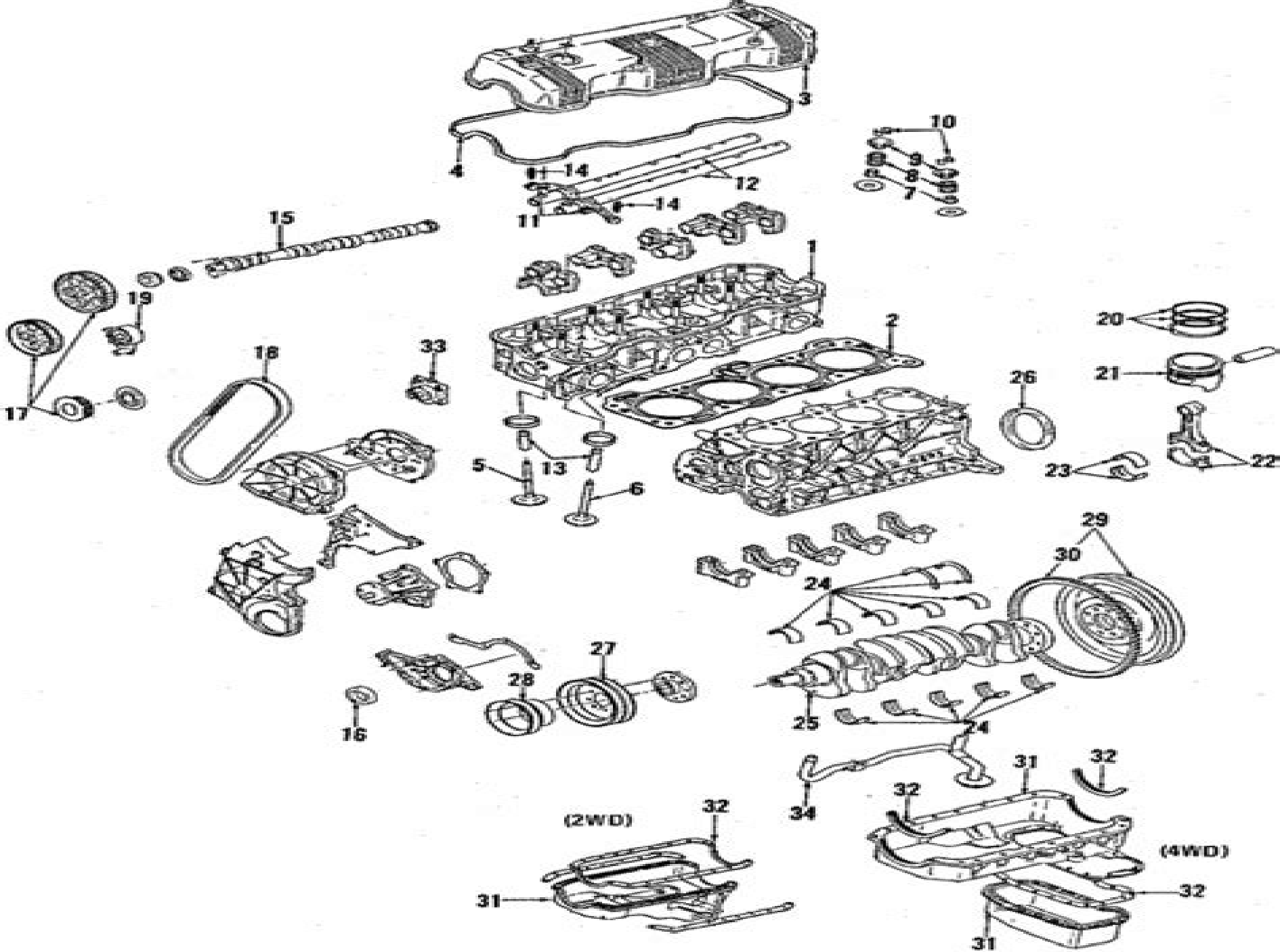
ENGINE — 2200CC/2300CC — GAS
