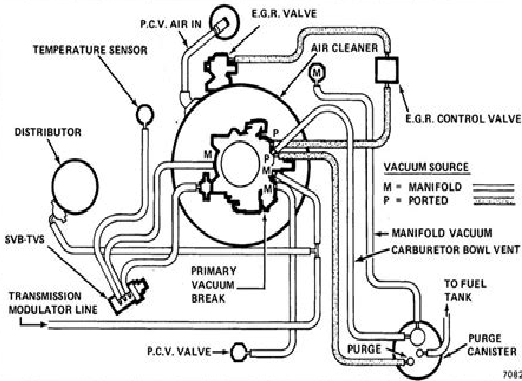
Fig. 6E-21 V8-403 488L VIN Code K Low Altitude
