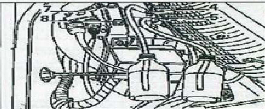
Purga del circuito de frenos. 4, 5, 7 y 8. Tornillos de purga del bloque hidráulico.
