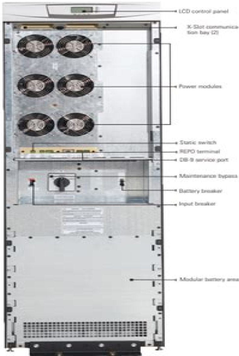
20/30 kVA UPS
