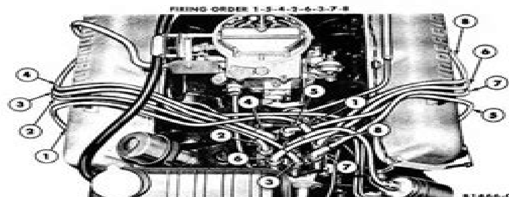
FIG. 26—Ignition Wiring
