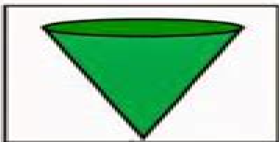
Cone
