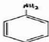
Anilina
