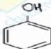
Fenolo
