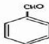
Benzaldeide
