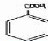
Ac. benzoico
