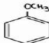
Anisolo
