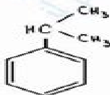
Cumene
