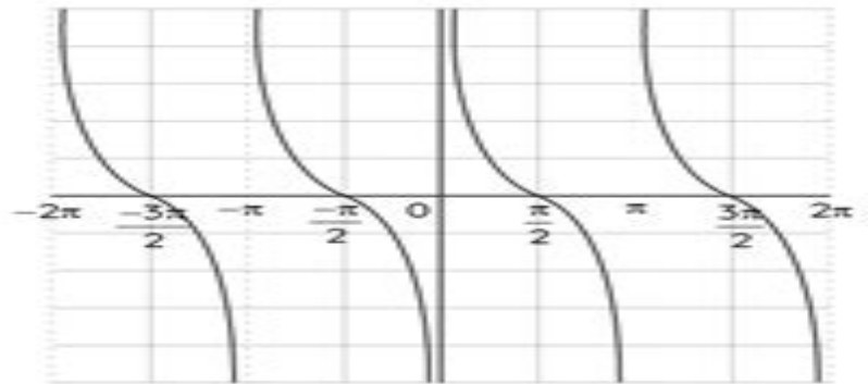
\cot\theta
