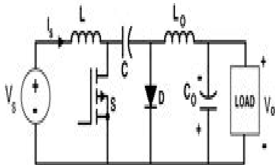
Cuk Converter
