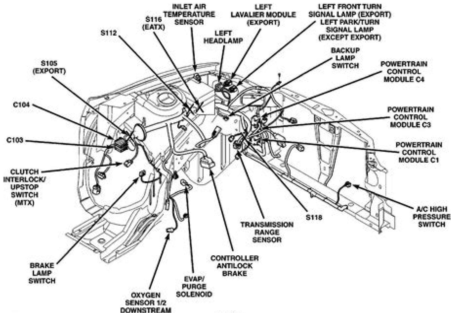
VIEW Y
